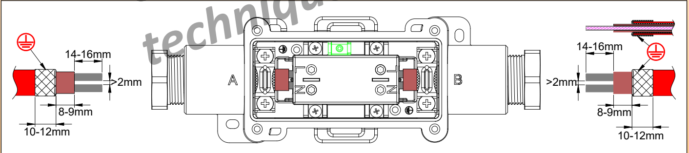
Modèle à deux câbles chauffants
