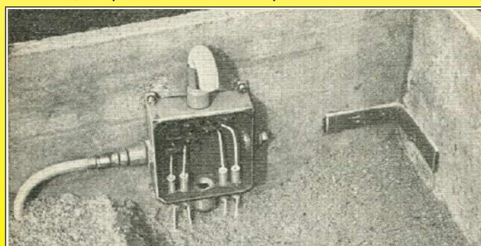
Chauffage électrique du sol, vue de l'arrivée des câbles chauffants (1957, Manuel EDF, Musée Ultimheat*)
