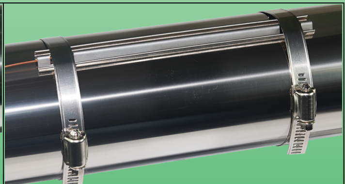
Exemple du modèle pour bulbe de thermostat après installation
