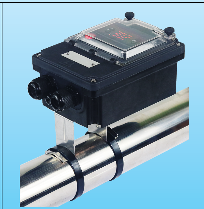
Exemple de montage avec l'option platine arrière de montage sur tube vertical
