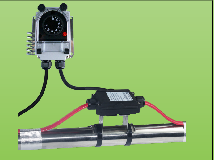
Exemple de montage en commande de deux câbles chauffants pour mise hors gel d'un tuyau en acier, combiné avec un boîtier Y27.
